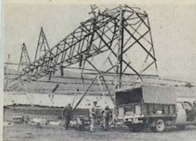
Una cuadrilla de 25 hombres trabajaba ayer en Coronel en la reparación de las torres de alta tensión derribadas por cargas explosivas. Mientras tanto, Carabineros seguía man-
